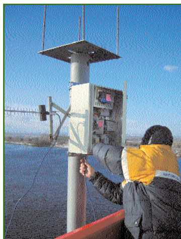
Рис. 11 Монтаж блока аппаратуры системы мониторинга моста через р. Енисей вблизи Красноярска
